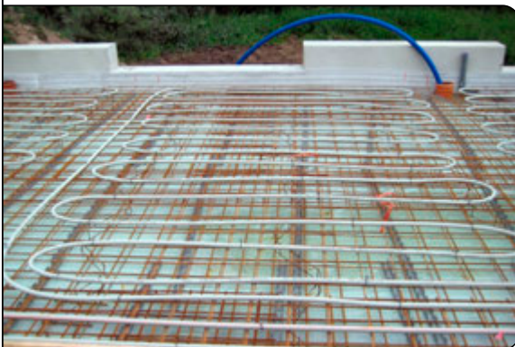
Rohrbefestigung an den Baustahlmatten
